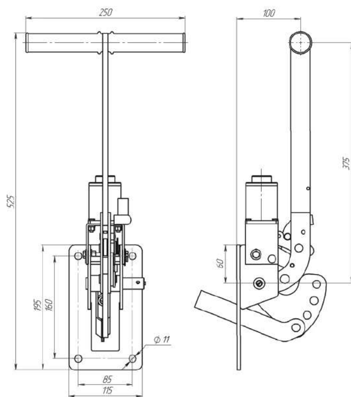
Габаритные и установочные размеры привода ПРА-17
