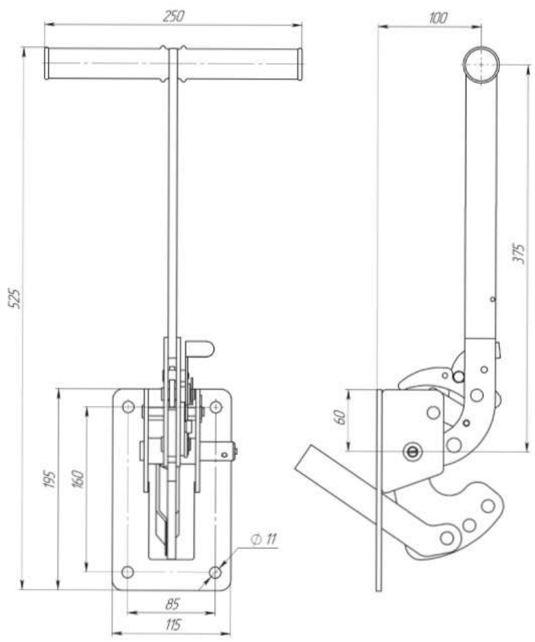
Габаритные и установочные размеры привода ПР-17
